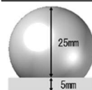
Fig.3 突起の大きさ Size of protrusion
